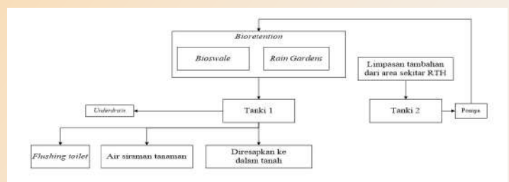
Gambar 1. Usulan konsep sistem sirkulasi hidrologi di RTH
